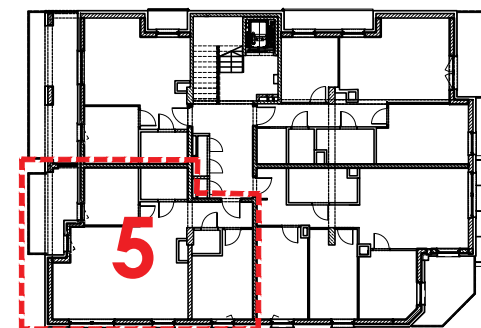
schemat kondygnacji
